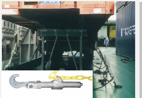
Kettenverzurrung
