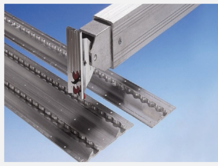
Gelenkladebalken 1841 und 1841 HD Aluminiumführungsschienen 5050 und 5052
