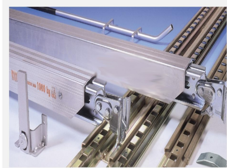
Gelenkladebalken 1840 und 1840 HD Stahlführungsschienen 5044 und 5046
