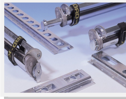
Kleiderstangen für Schiene 1806 Schiene 1803 Schiene 3009/2010
